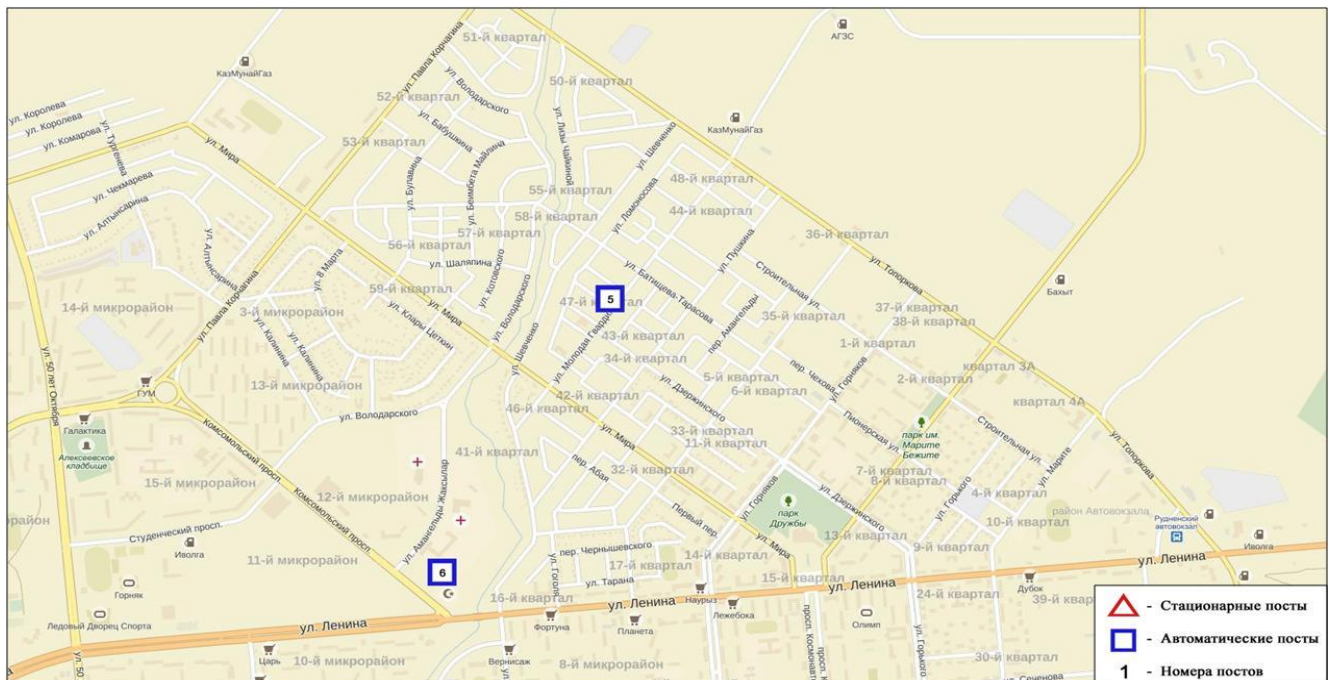
Схема расположения стационарной сети наблюдения за загрязнением атмосферного воздуха города Рудный
