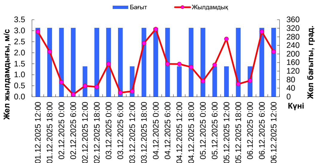
21050 квадратындағы жел жағдайлары
