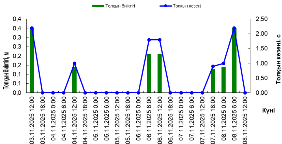
21050 квадратындағы толқындар
