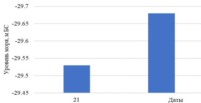
Рисунок. График хода изменения уровня моря в Фетисово 21 августа 2025 г.
