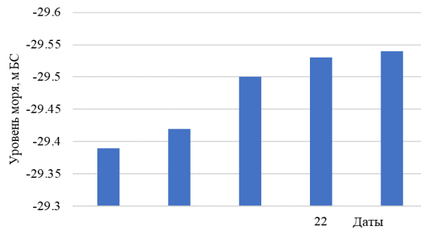
Рисунок. График хода изменения уровня моря в Фетисово 21-22 августа 2025 г.
