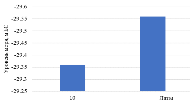
Рисунок. График хода изменения уровня моря в Фетисово 10 августа 2025 г.
