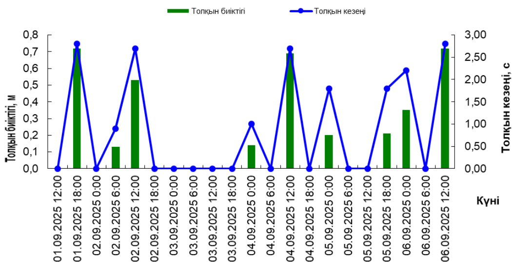
21050 квадратындағы толқындар
