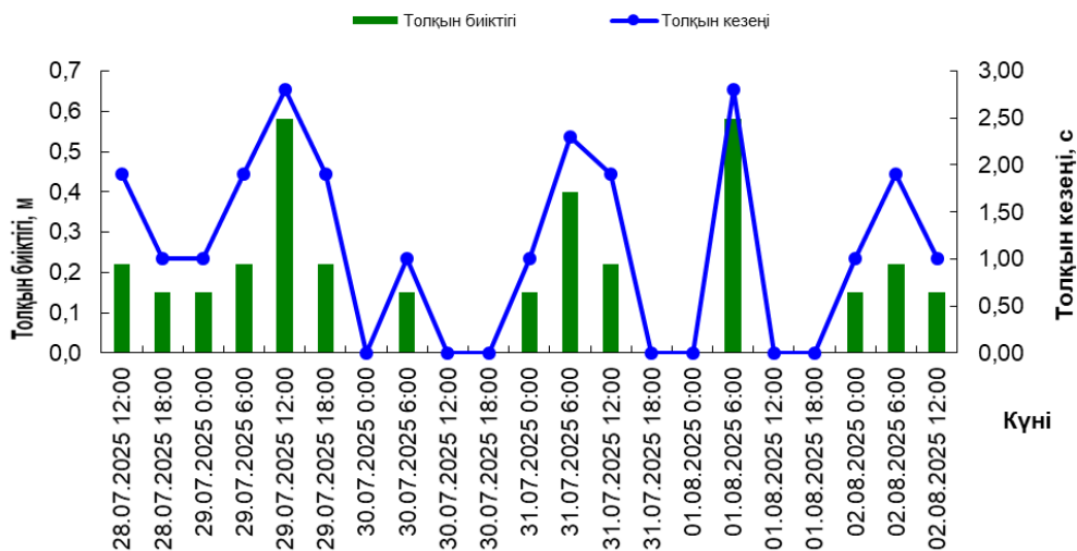
21050 квадратындағы толқындар
