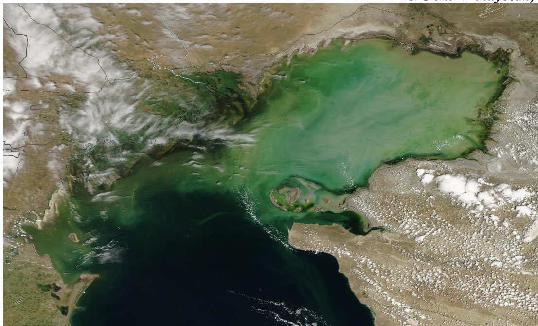
1-сурет. 2025 ж. 26 маусымдағы ғарыштан түсірілген Каспий теңізінің NASA/GSFC фотосуреті
