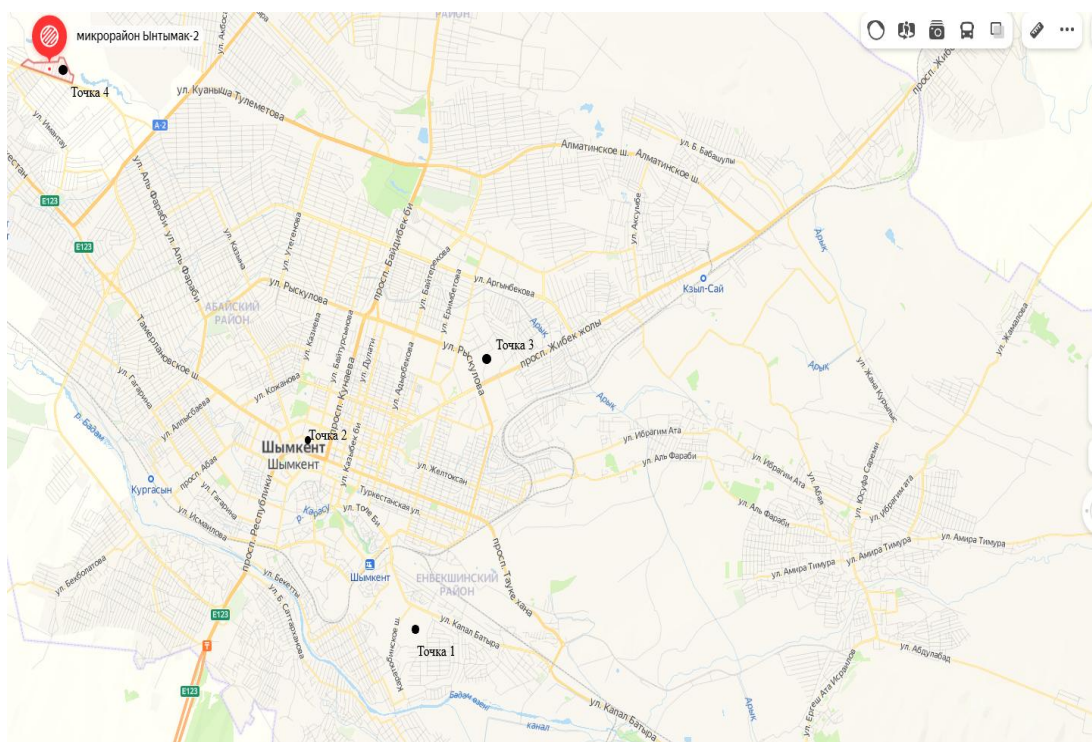
Сурет 2 - Шымкент қ. атмосфералық ауаның ластануын бақылаудың экспедиционный желісінің орналасу схемасы
