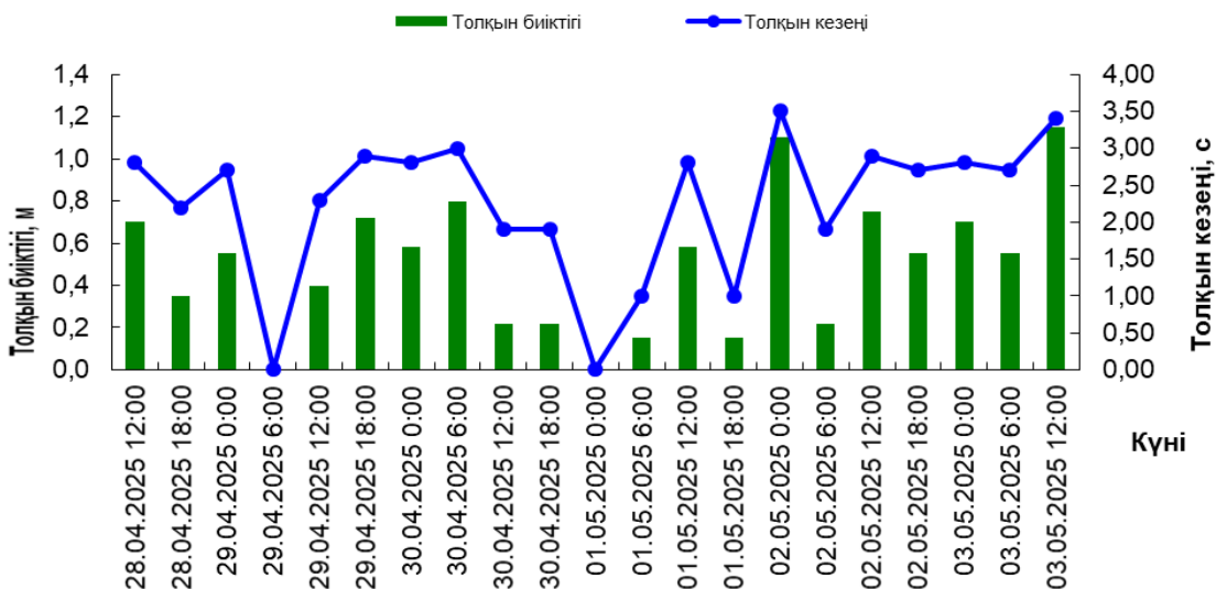
21050 квадратындағы толқындар
