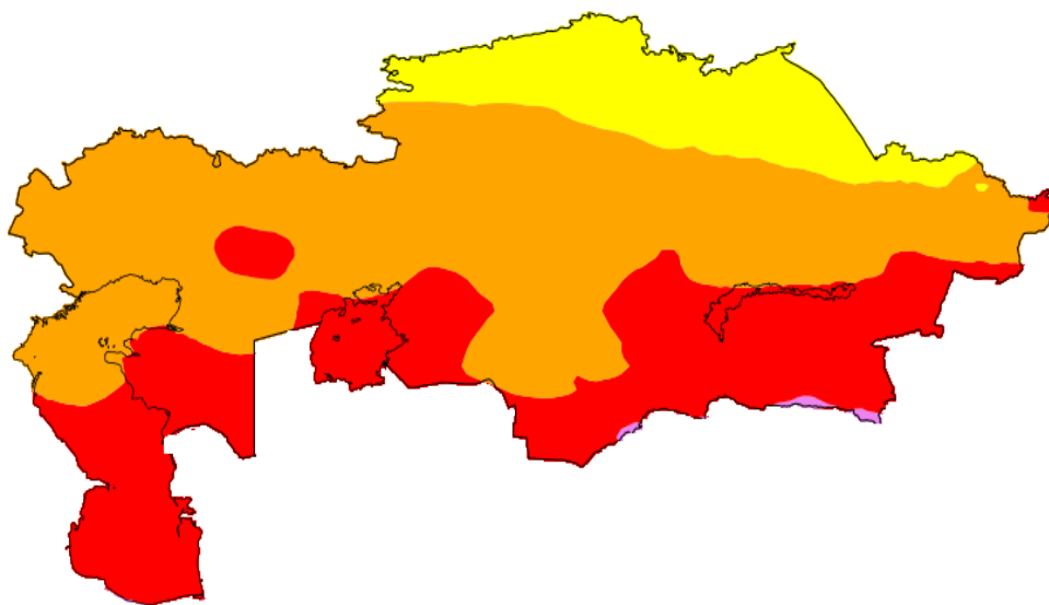
Рис. Распределение УФ индекса по территории Казахстана 28 мая 2021 г.
