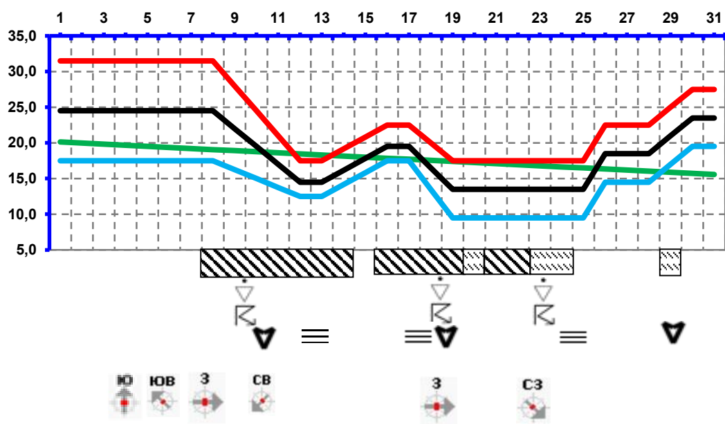
График хода погоды в августе
