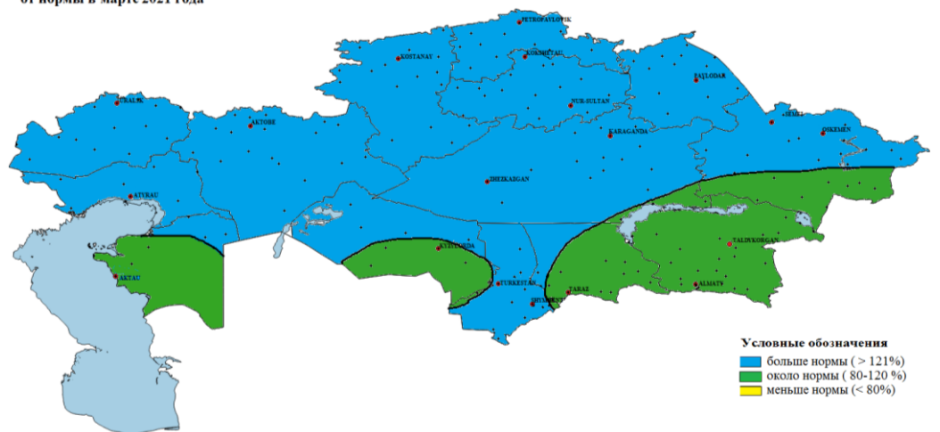
Ожидаемые отклонения количества осадков от нормы в марте 2021 года
