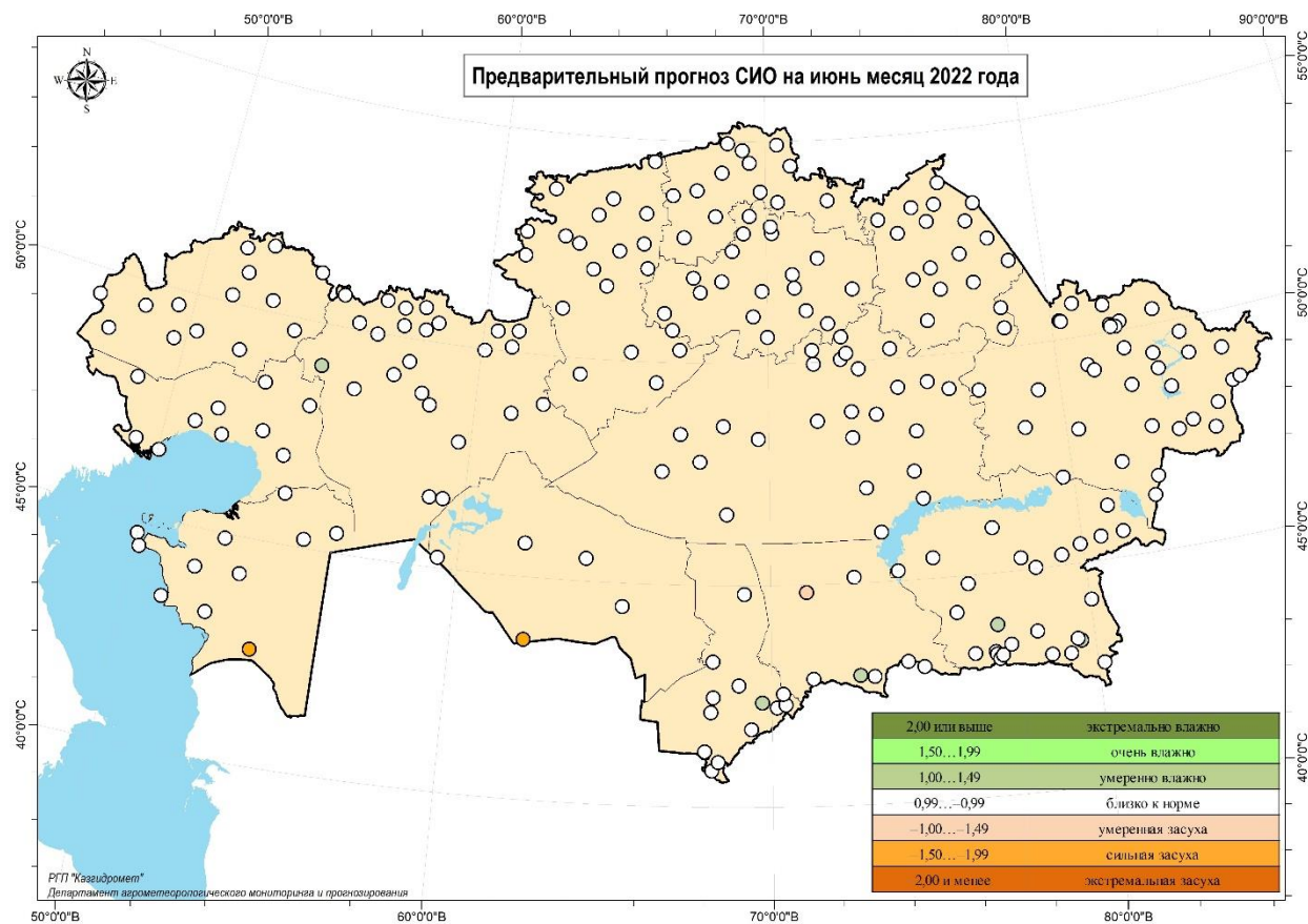
1-сурет. Жауын-шашынның стандартталған индексінің (ЖСИ_1) мәндері негізіндегі Қазақстан аумағының ылғалдану жағдайларының 2022 жылдың маусым айына арналған статистикалық алдын ала болжамы.
