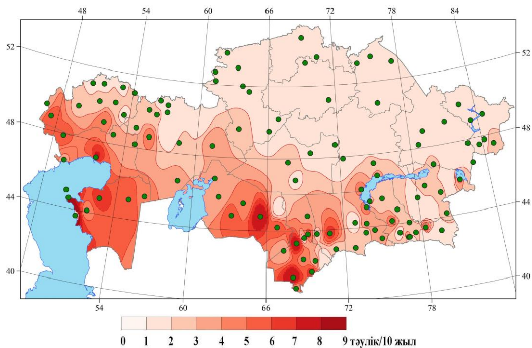
2.26 – сурет. 1961–2024 жж. кезеңіндегі тропикалық түндер (тәулік/10 жыл) санының өзгеру қарқыны (TR индексі)
