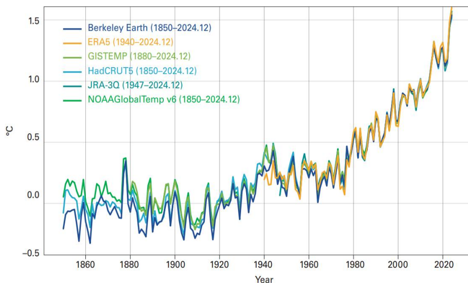
1.1-сурет. Орташа жаһандық температураның жылдық аномалиялары индустрияға дейінгі кезеңмен (1850–1900 жж.) салыстырғанда 1850 жылдан 2024 жылға дейінгі аралықта көрсетілген.
