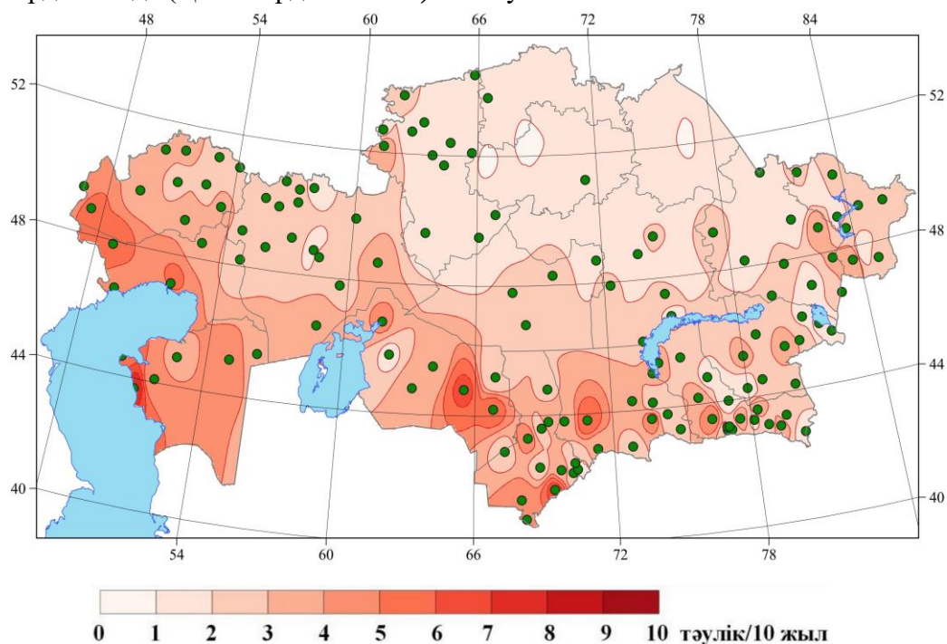
2.21 – сурет. 1961-2024 жж. кезеңіндегі жылы кезеңде (тәулік/10 жыл) жылу толқындарының жалпы ұзақтығының өзгеру қарқыны (HWF/ENF индексі)
