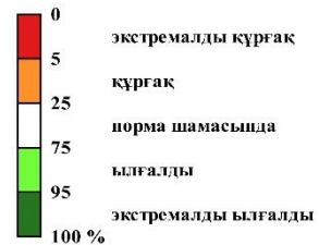
3.1-сурет. 2024 жыл үшін норма % бойынша көрсетілген жылдық және мезгілдік жауын-шашын мөлшері (сол жақта), сондай-ақ 1961–2024 жылдар кезеңіне есептелген оның асып кетпеу ықтималдығының (оң жақта) географиялық таралуы. 1-парақ
