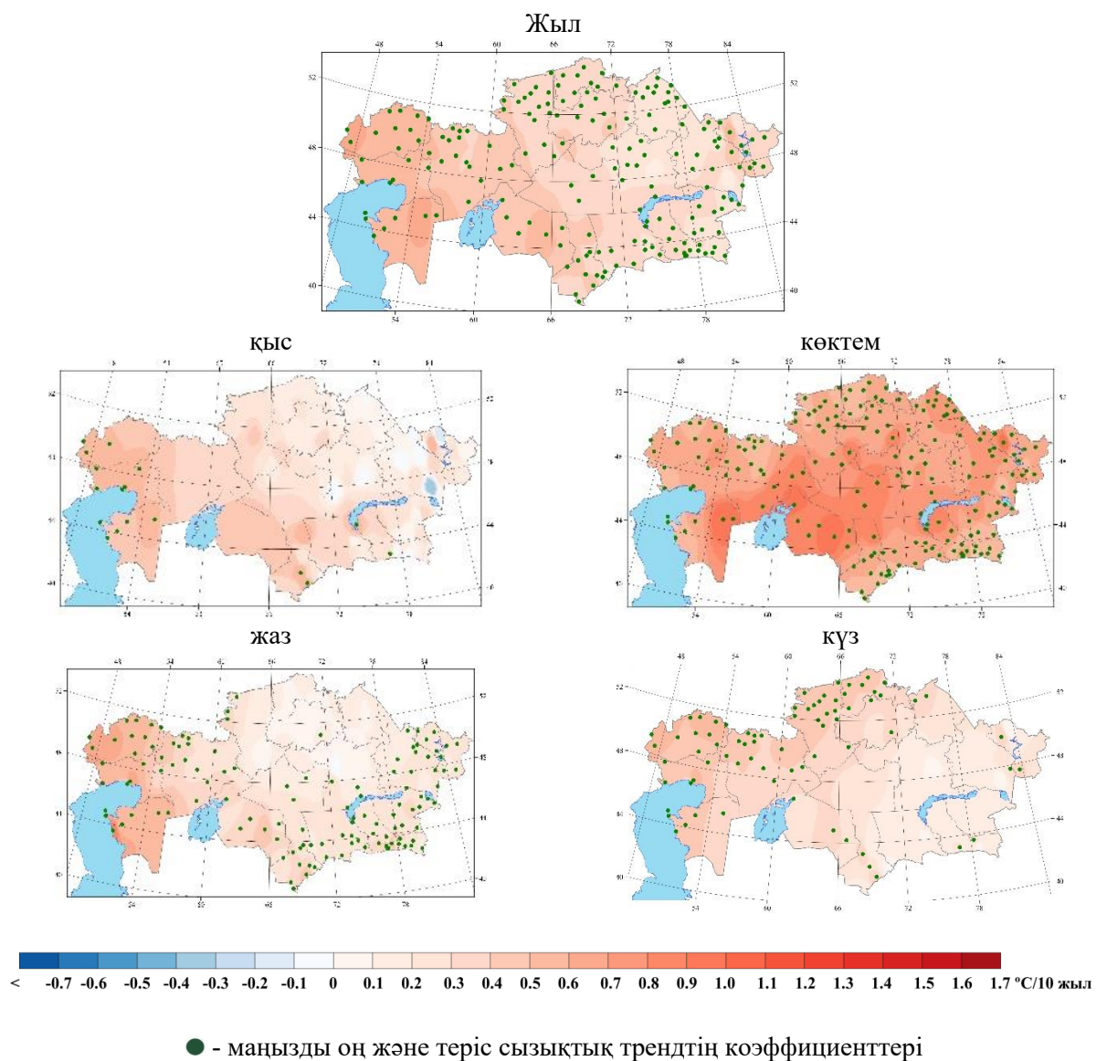
2.16 сурет. 1976–2024 жж. кезеңінің бақылау деректері бойынша есептелген орташа жылдық және мезгілдік жер беті ауа температурасының (°C/10 жыл) сызықтық тренд коэффициенттері мәндерінің кеңістіктік таралуы.
