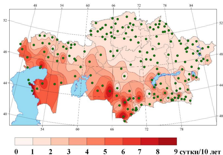
Рисунок 2.26 – Темпы изменения количества тропических ночей (сутки/10лет) в период 1961–2024 гг. (индекс TR)
