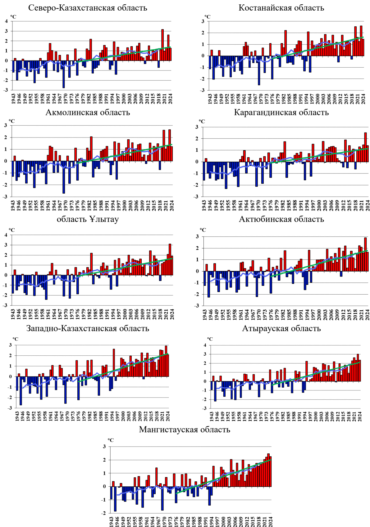
Рисунок 2.15 – Временные ряды аномалий годовых температур воздуха ( ^{\circ}\text{C} ), осредненных по областям Казахстана за период 1941–2024 гг. Аномалии рассчитаны относительно базового периода 1961–1990 гг. Линейный тренд за период 1976–2024 гг. выделен зеленым цветом. Сглаженная кривая получена 11-летним скользящим осреднением. Лист 2
