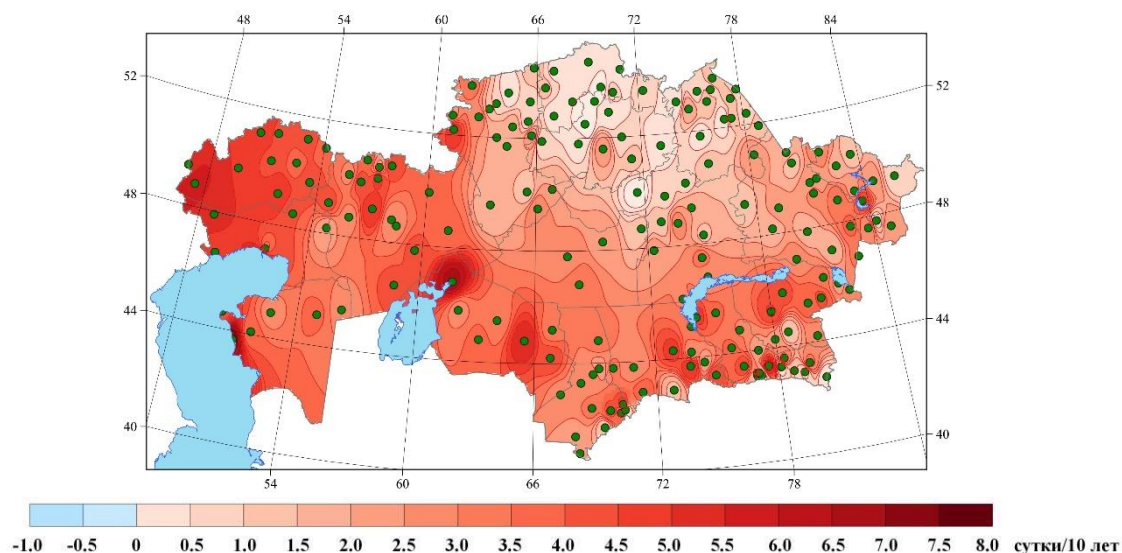
Рисунок 2.20 – Темпы изменения количества суток, когда максимальная суточная температура равна или выше 30 °C (сутки/10 лет) в период 1961–2024 гг. (индекс TХ_{де30} )
