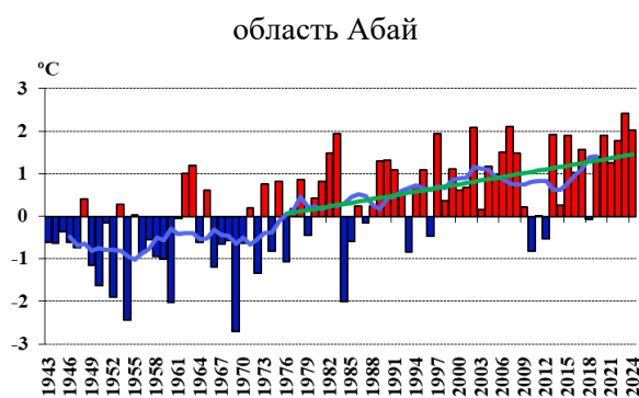
Рисунок 2.15 – Временные ряды аномалий годовых температур воздуха (°C), осредненных по областям Казахстана за период 1941–2024 гг. Аномалии рассчитаны относительно базового периода 1961–1990 гг. Линейный тренд за период 1976–2024 гг. выделен зеленым цветом. Сглаженная кривая получена 11-летним скользящим осреднением. Лист 1
