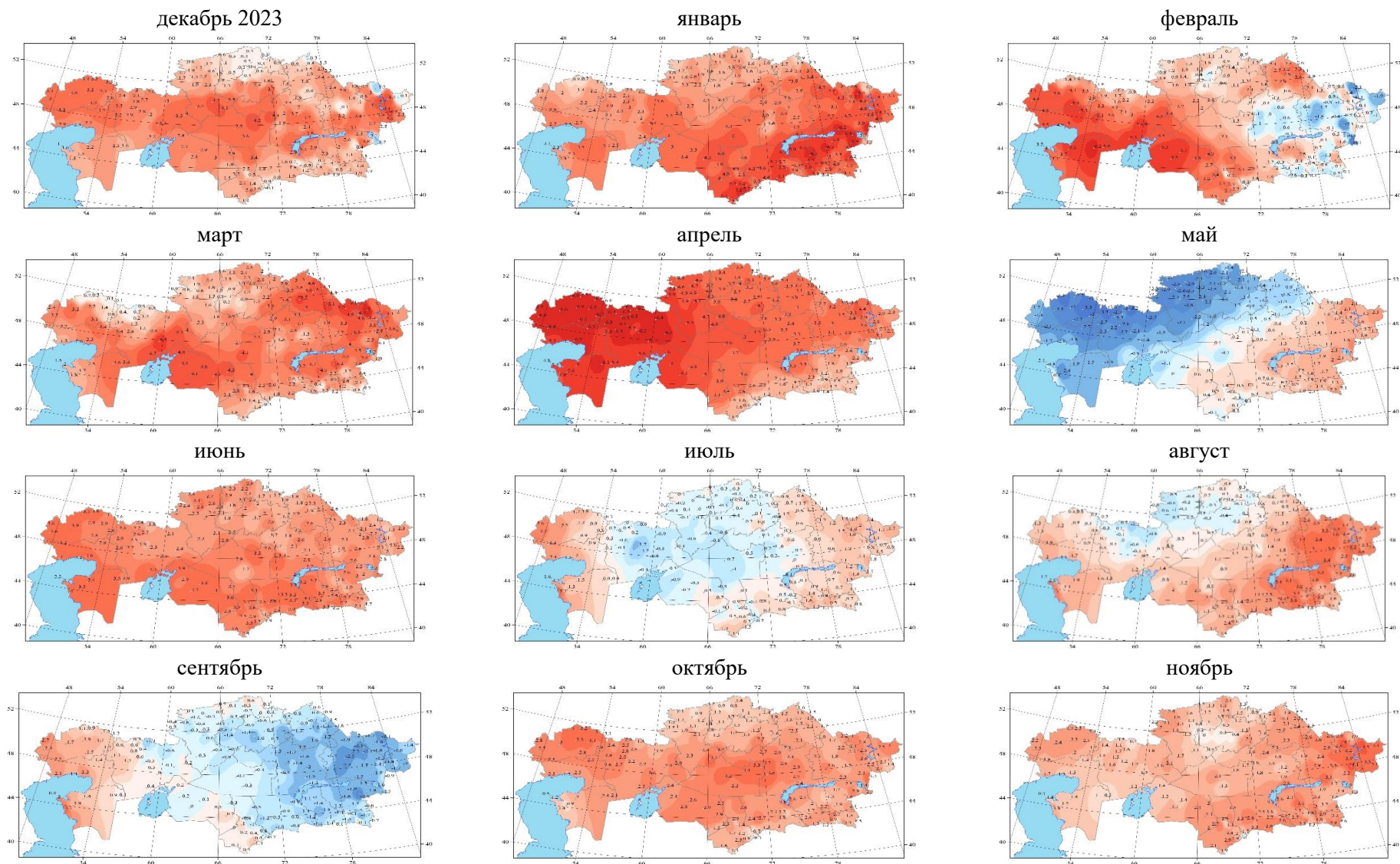
Рисунок 2.5 – Пространственное распределение аномалии среднемесячной температуры воздуха ( ^{\circ}\text{C} ) в 2024 году, рассчитанных относительно базового периода 1961–1990 гг.
