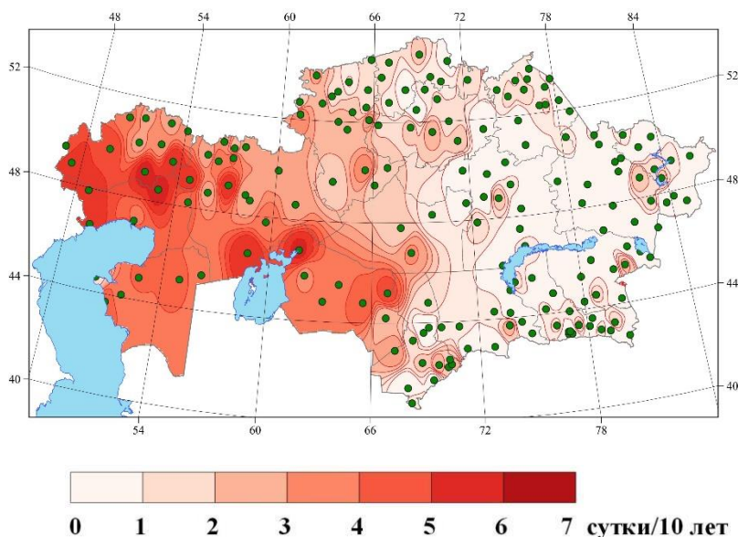
Рисунок 2.24 – Темпы изменения общей за год продолжительности волн тепла (сутки/10лет) в период 1961–2024 гг. (индекс WSDI)
