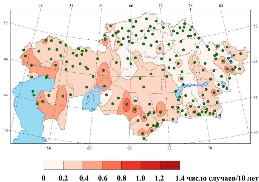
Рисунок 2.22 – Темпы изменения количества волн жары в теплый период (число случаев/10лет) в 1961–2024 гг. ( индекс HWN )
