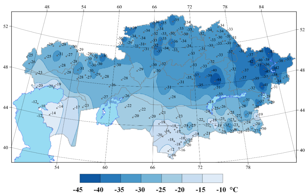
Рисунок 2.12 – Значения суточной минимальной температуры воздуха (°C), зарегистрированные в 2024 г. (индекс TN_n )
