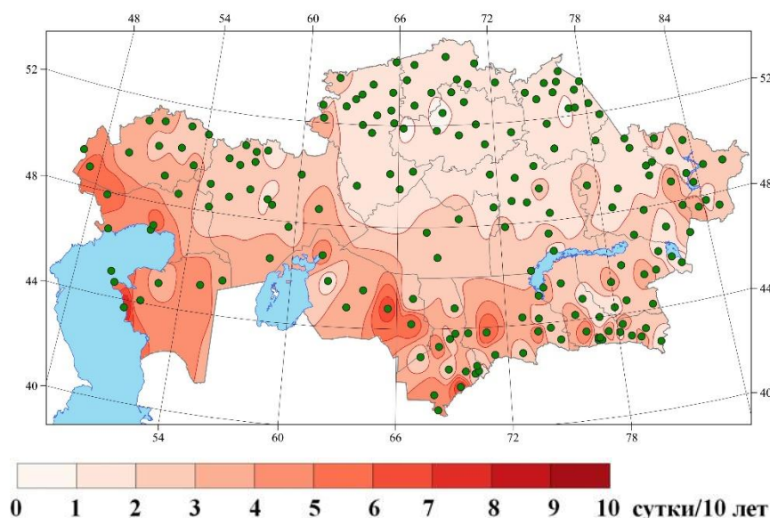
Рисунок 2.21 – Темпы изменения общей продолжительности волн тепла в теплый период (сутки/10лет) в 1961–2024 гг. (индекс HWF/EHF )
