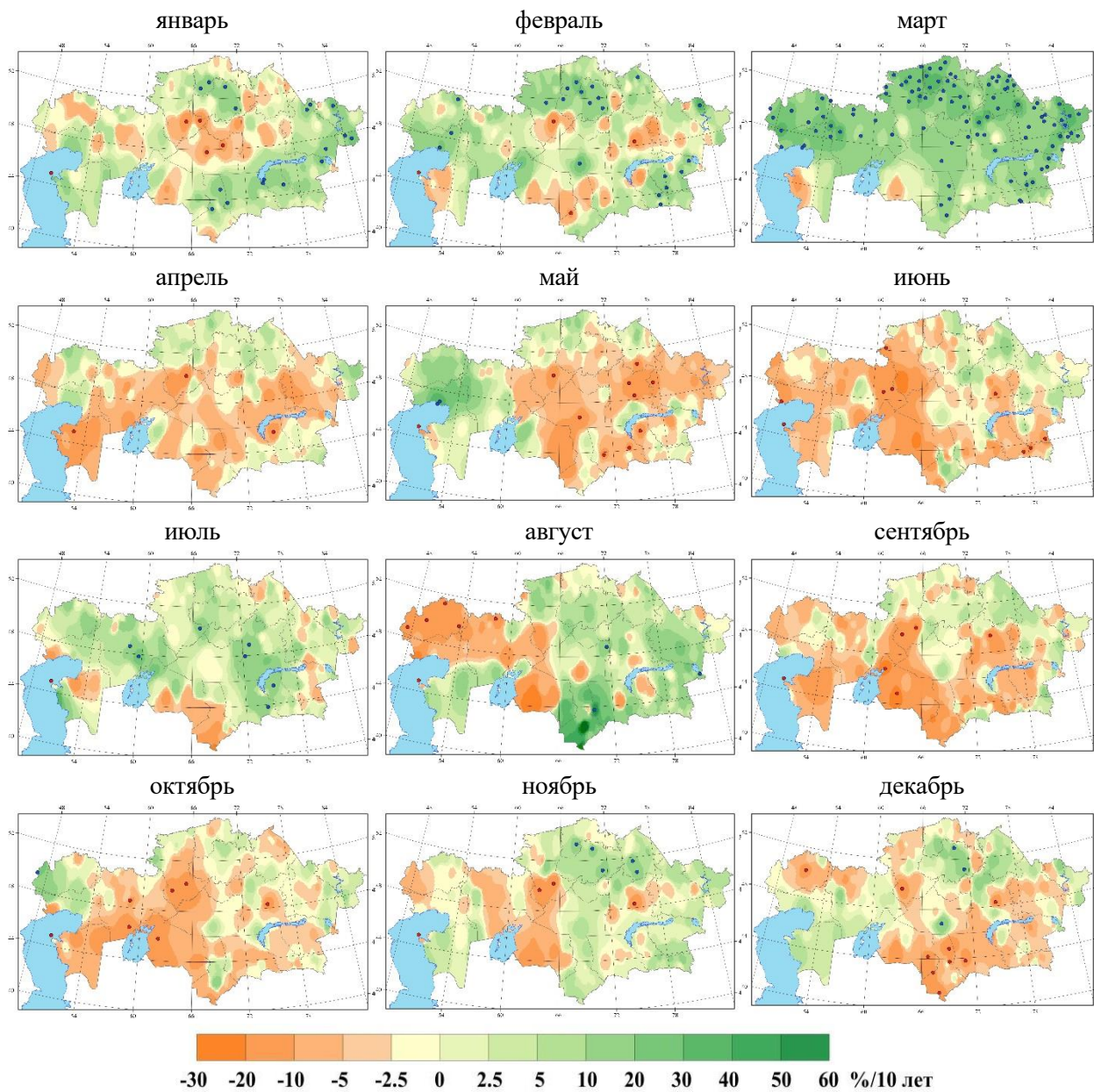
Рисунок 3.11 – Пространственное распределение значений коэффициента линейного тренда месячного количества осадков (%/10 лет), рассчитанного за период 1976 – 2024 гг.
