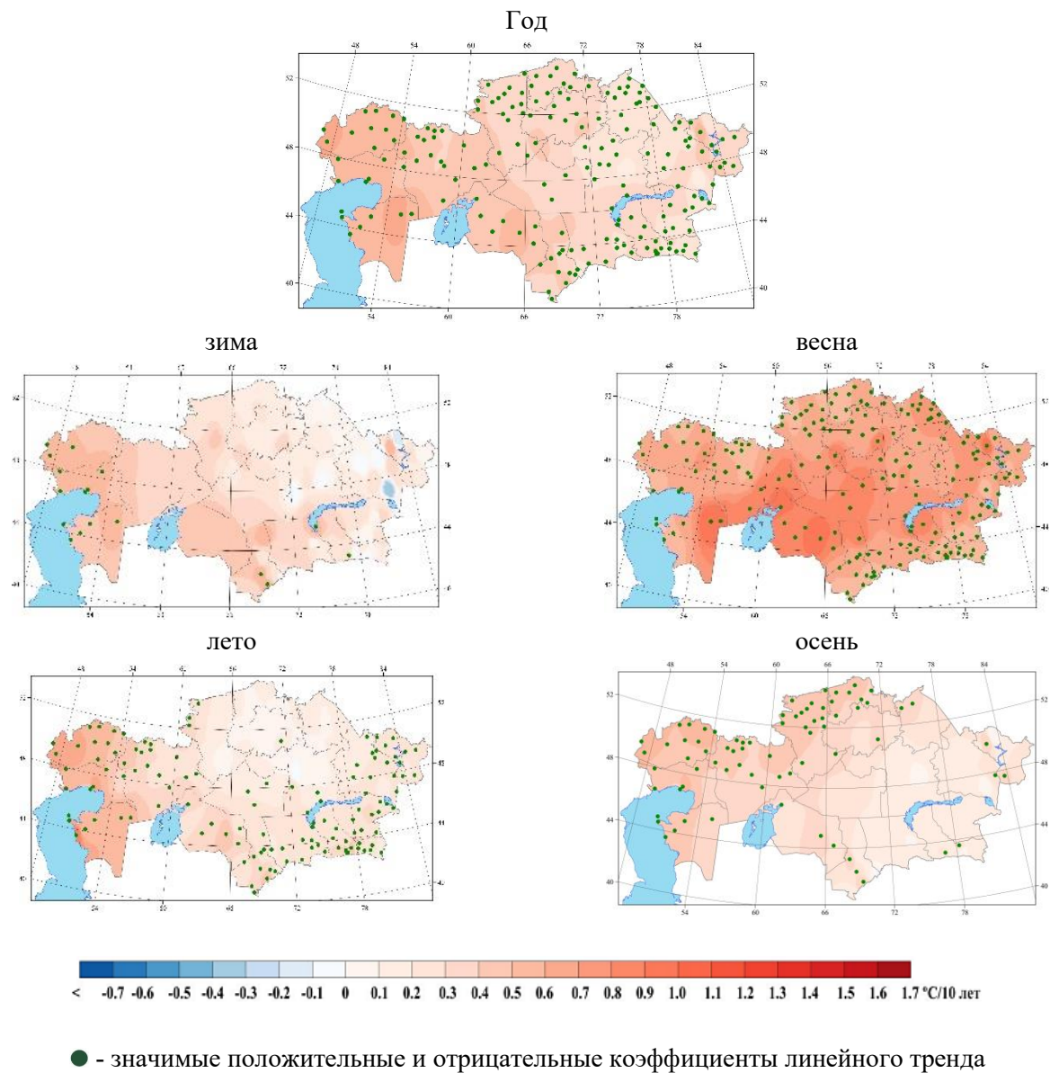
Рисунок 2.16 – Пространственное распределение значений коэффициента линейного тренда средней годовой и сезонной температуры приземного воздуха (°C/10 лет), рассчитанного по данным наблюдений за период 1976–2024 гг.
