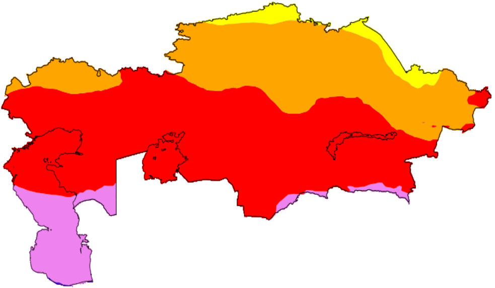
Рис. Распределение УФ индекса по территории Казахстана 29 мая 2020 г.
